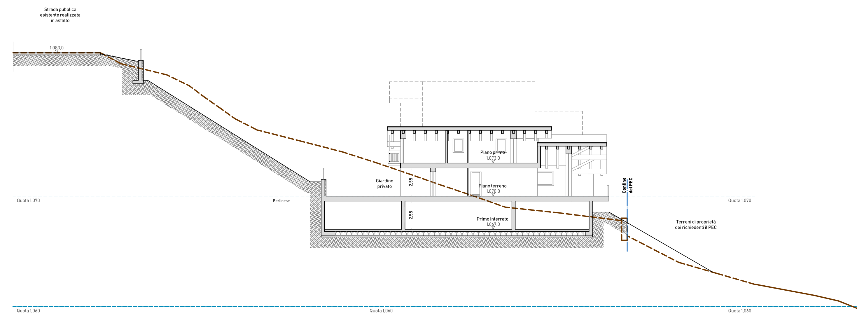
PROFILO 5-5 Scala 1:200
